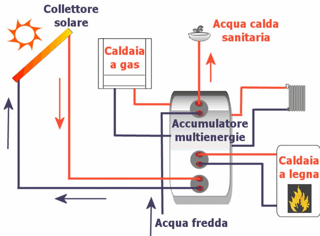
Kit circolazione forzata serie MULTI - Schema tecnico
